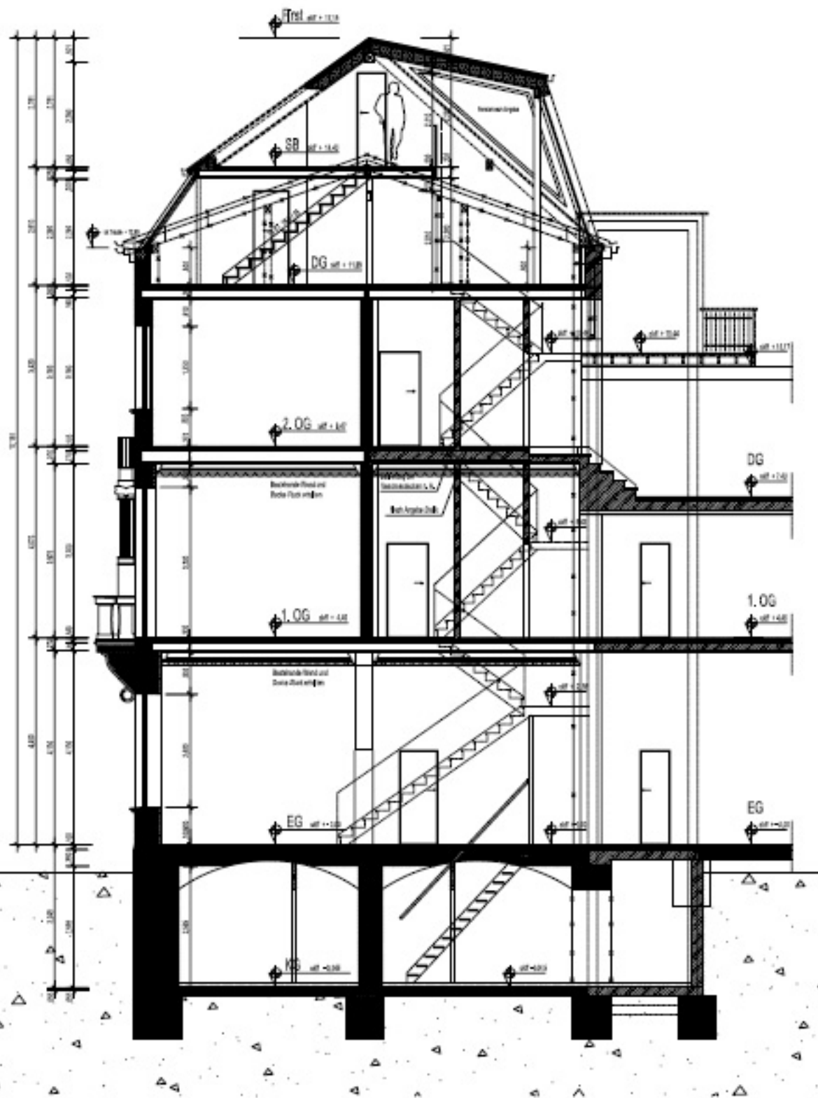
Schnitt B - B
