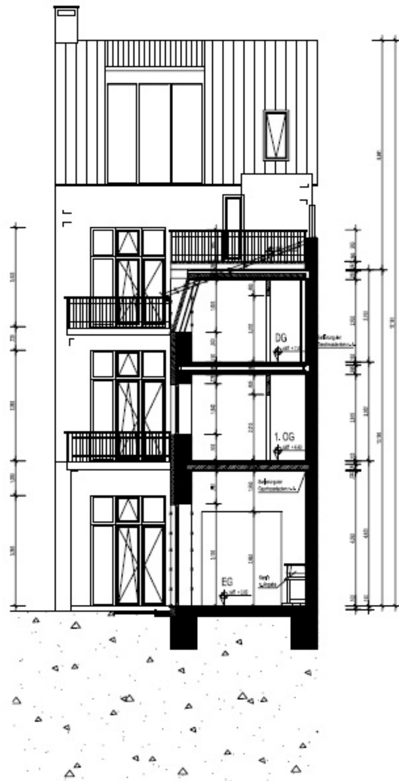
Schnitt C - C
